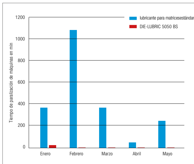
Tiempo de paralización de las máquinas causado por boquillas bloqueadas
